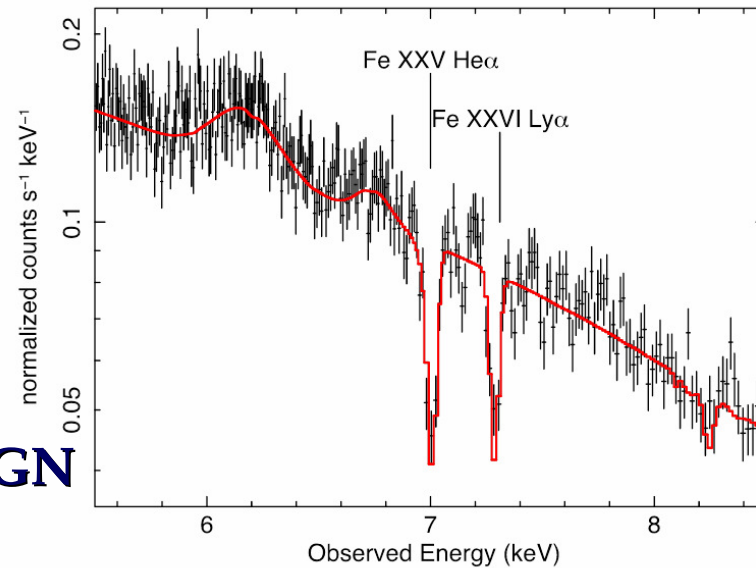
3C 120 Astro-H 100ks ( v_{\text{turb}}=1000\text{km/s} , Feb 2006)
